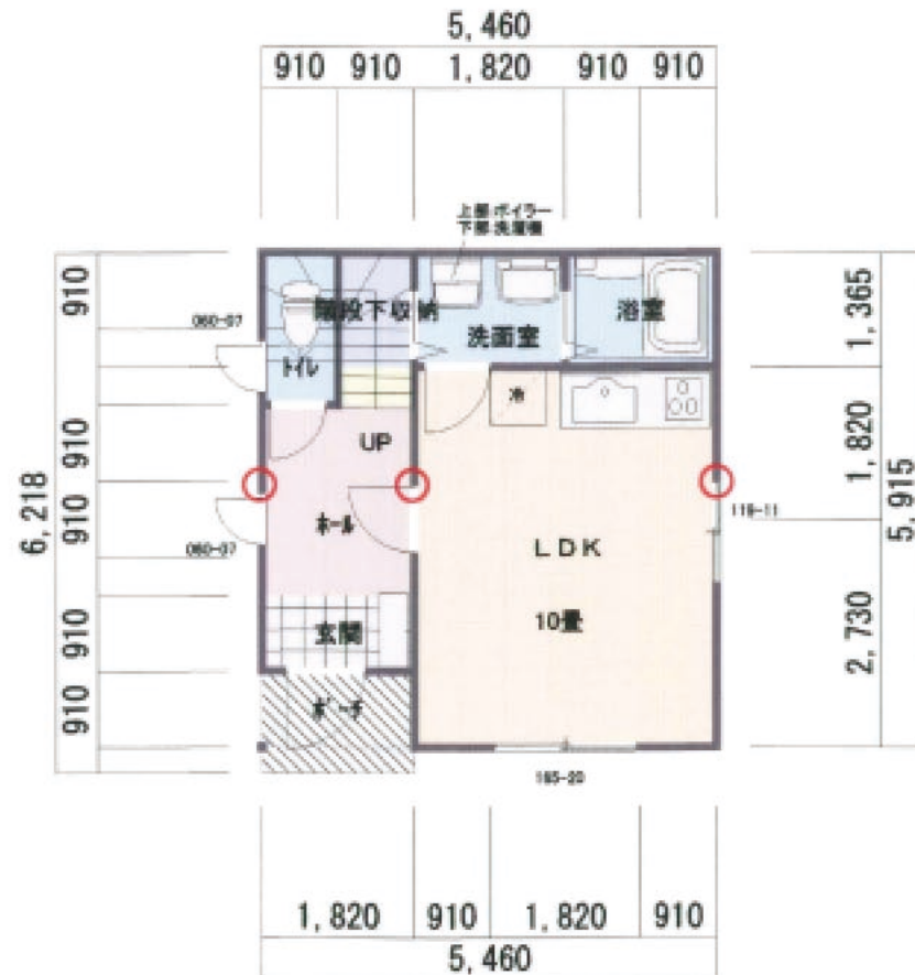
1階平面図
