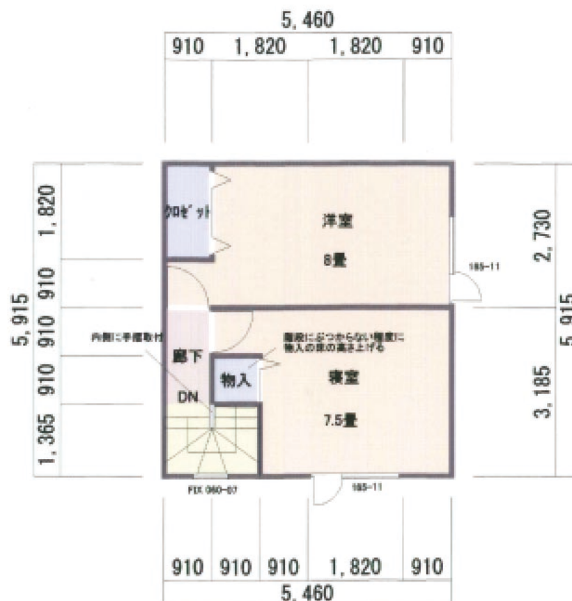
2階平面図
