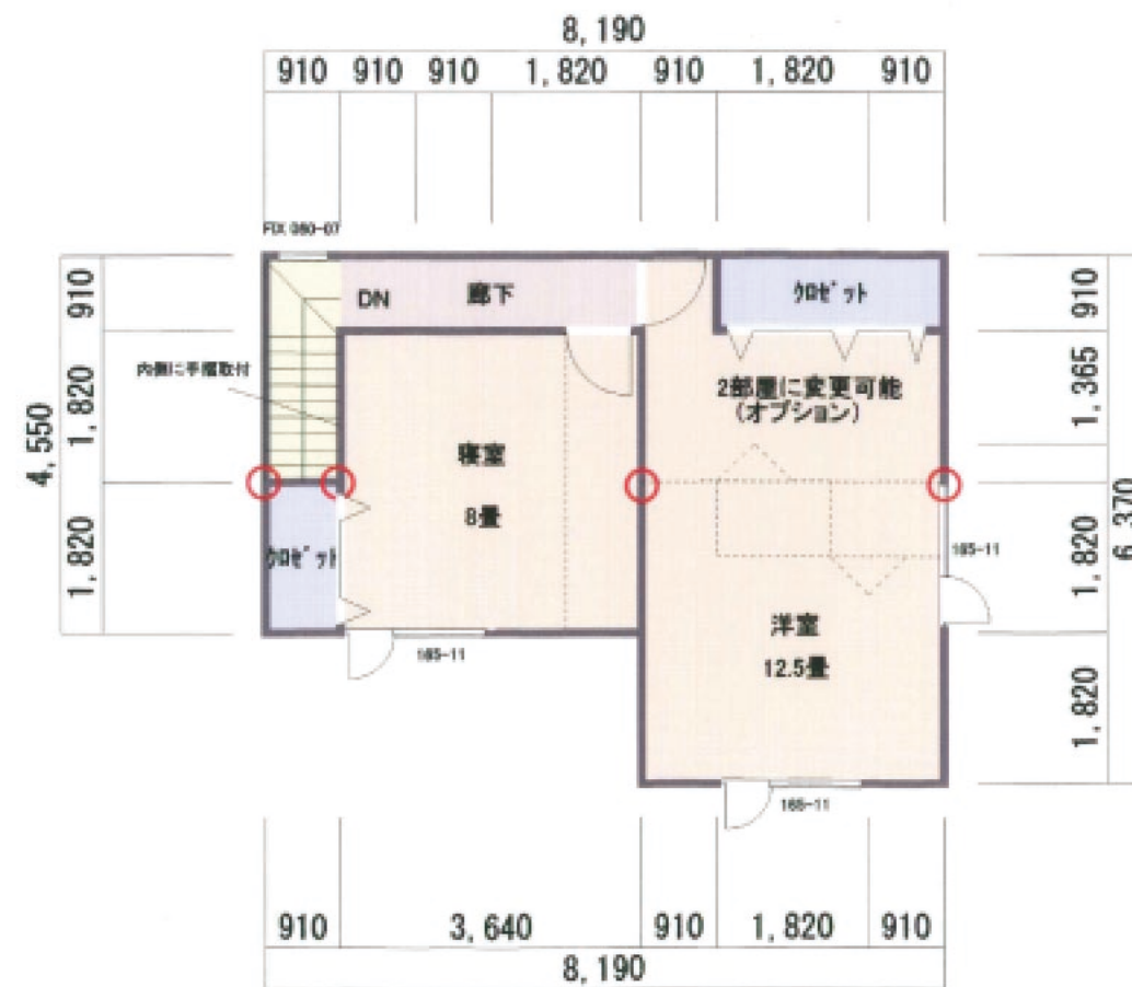
2階平面図
