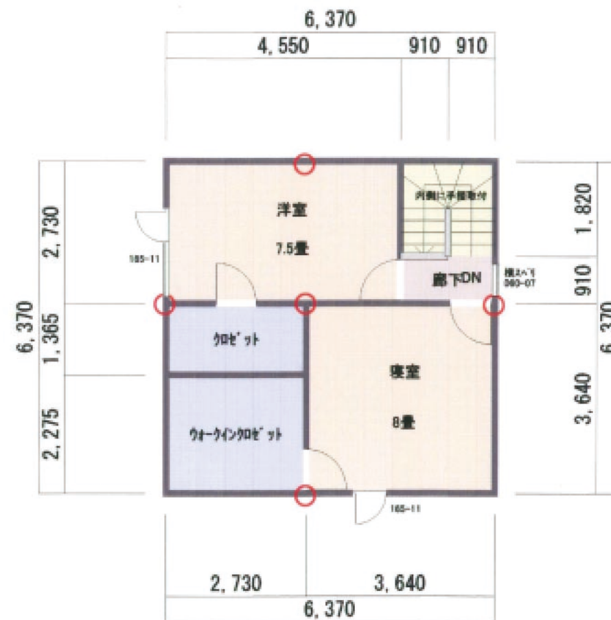
2階平面図
