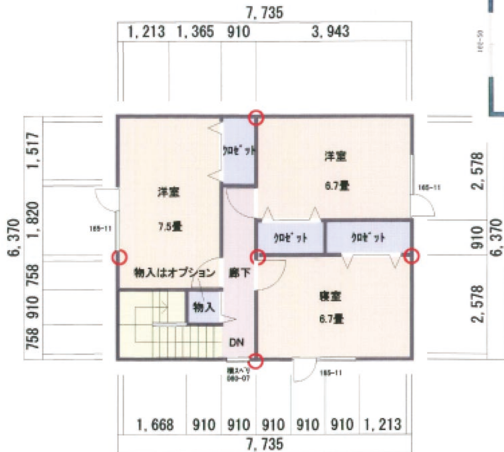
2階平面図
