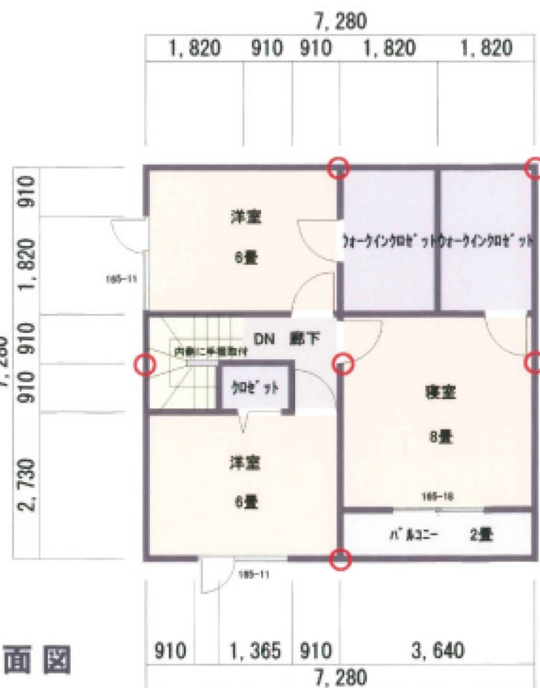
2階平面図
