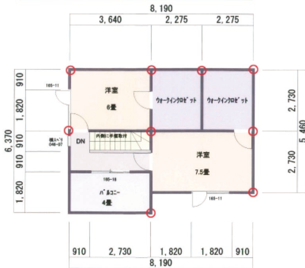
2階平面図
