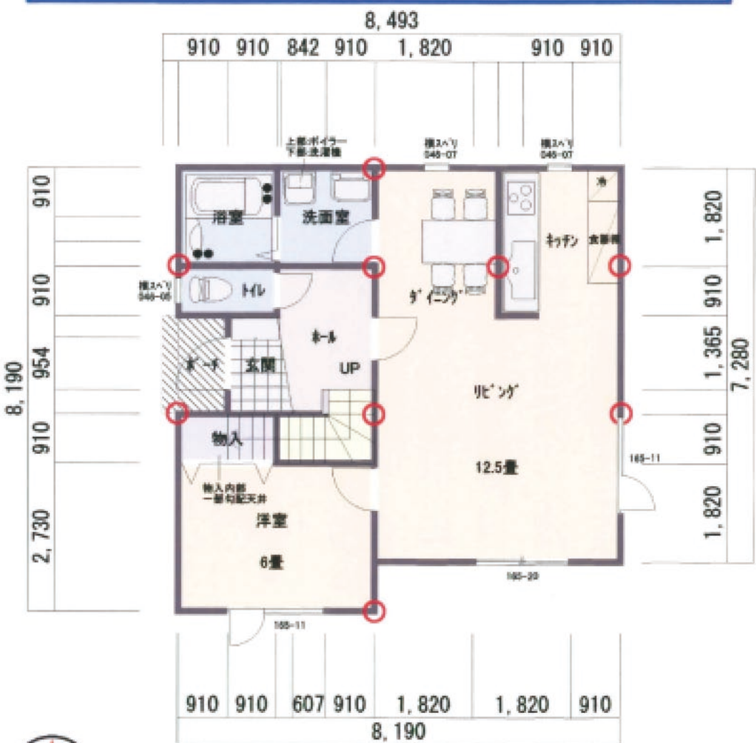
1階平面図
